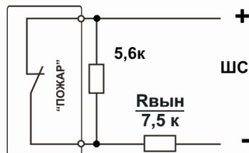
Рис. 14. Организация двухпорогового шлейфа пожарной сигнализации
