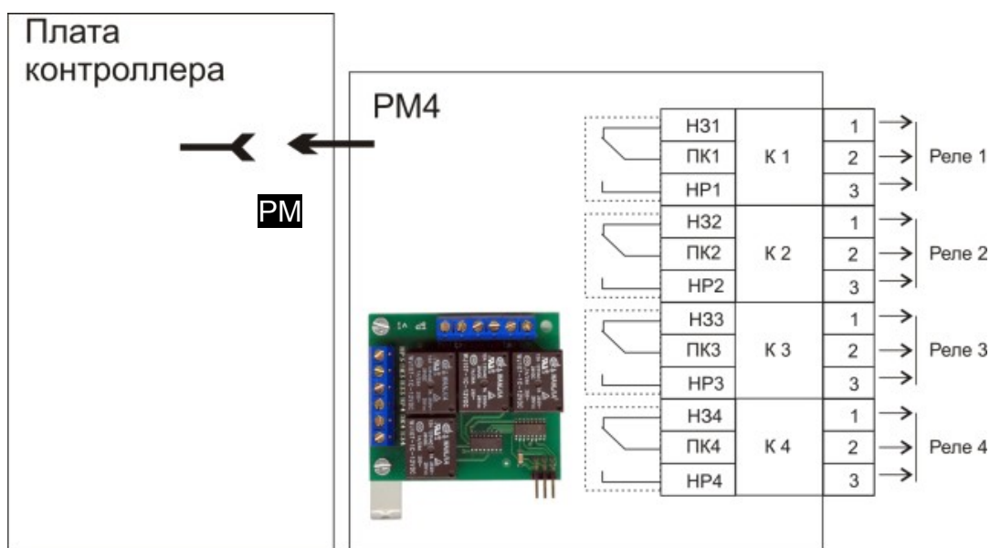
Рис. 8. Схема внешних подключений модуля реле.
