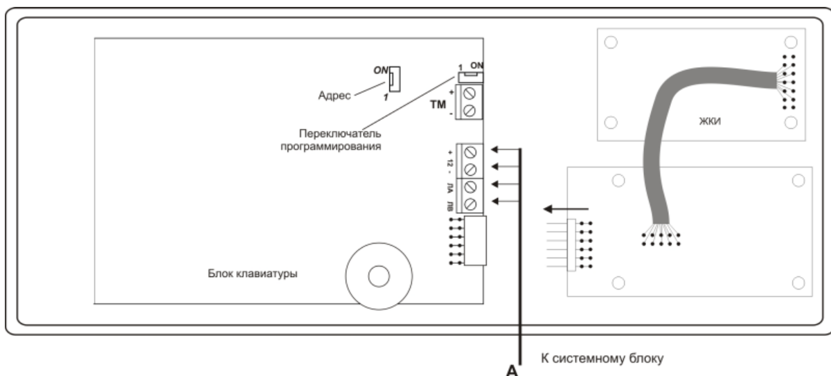
Рис. 7. Схема внешних подключений блока клавиатуры.
