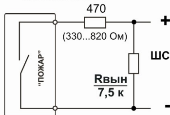
Рис. 14. Организация двухпорогового шлейфа пожарной сигнализации
