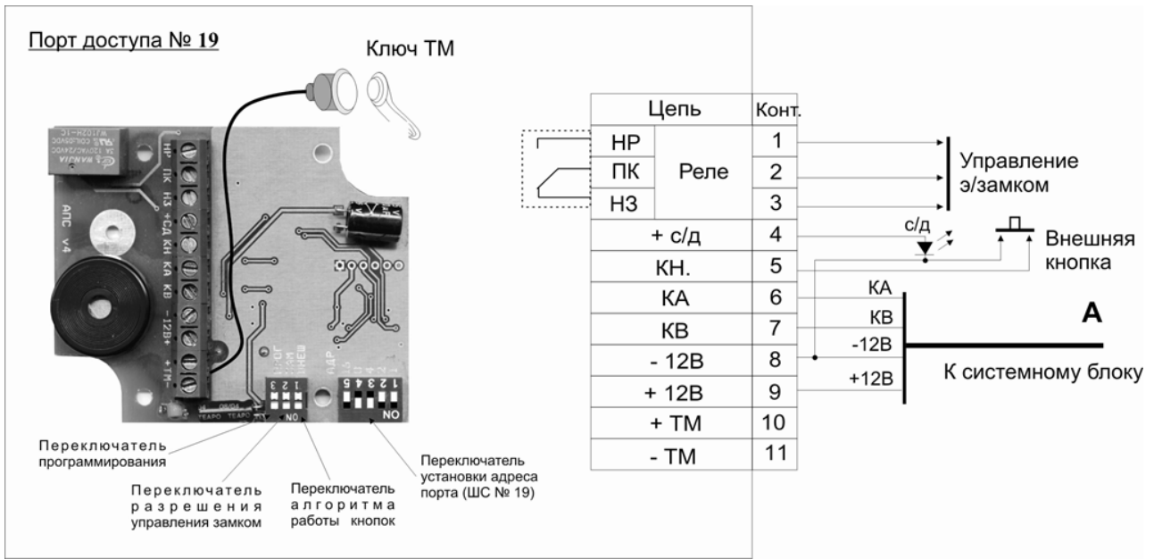
Рис. 11. Схема подключения порта доступа.
