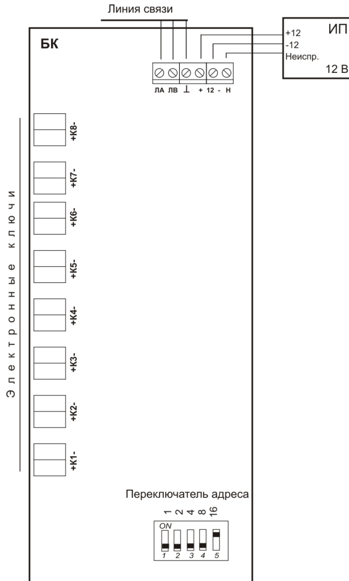
Рис. 10. Схема подключения блока ключей.
