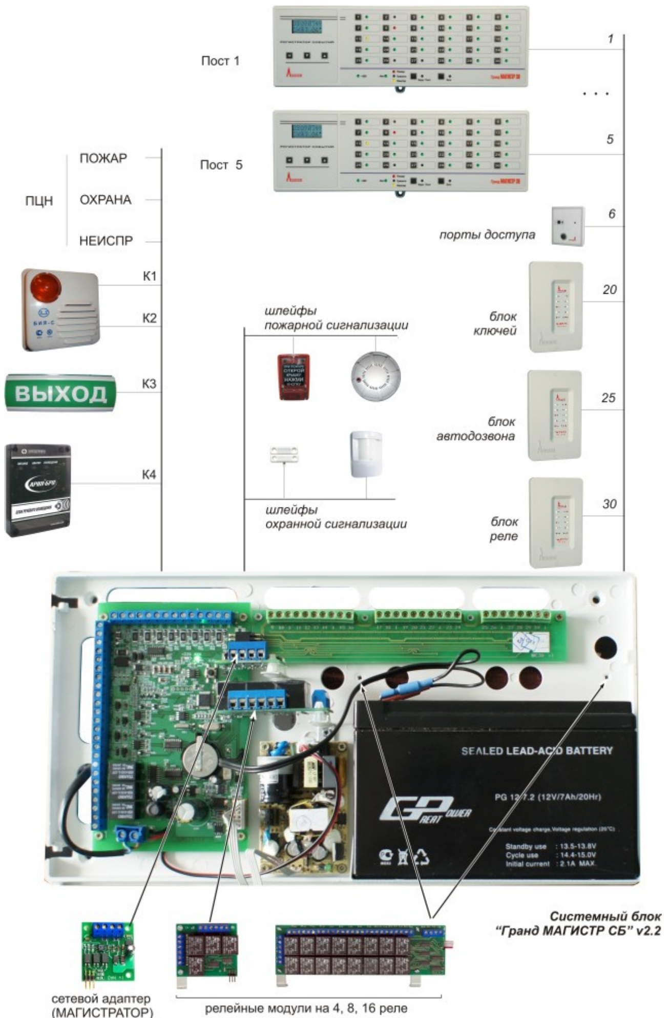
Рис. 1. Состав прибора «Гранд Магистр» (версия 2)
