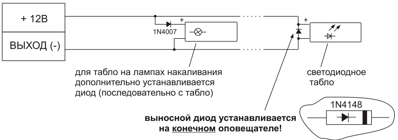
Рис. 17. Схема подключения нескольких световых табло
