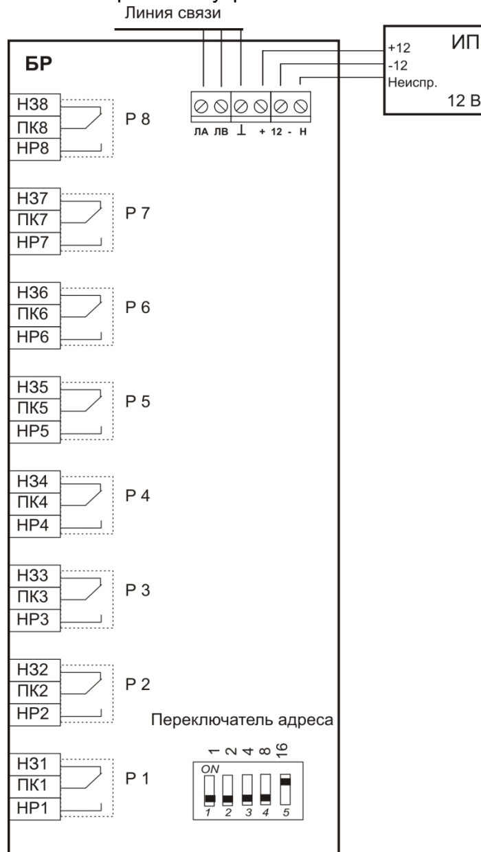
Рис. 9. Схема подключения блока реле.
