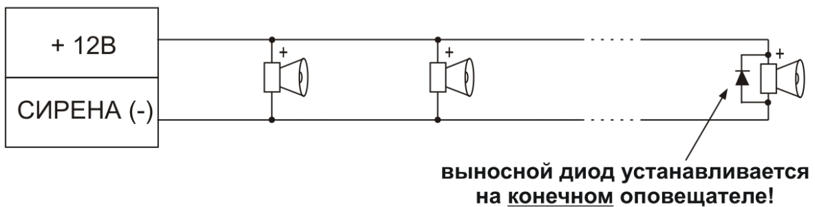
Рис. 18. Схема подключения нескольких звуковых оповещателей
