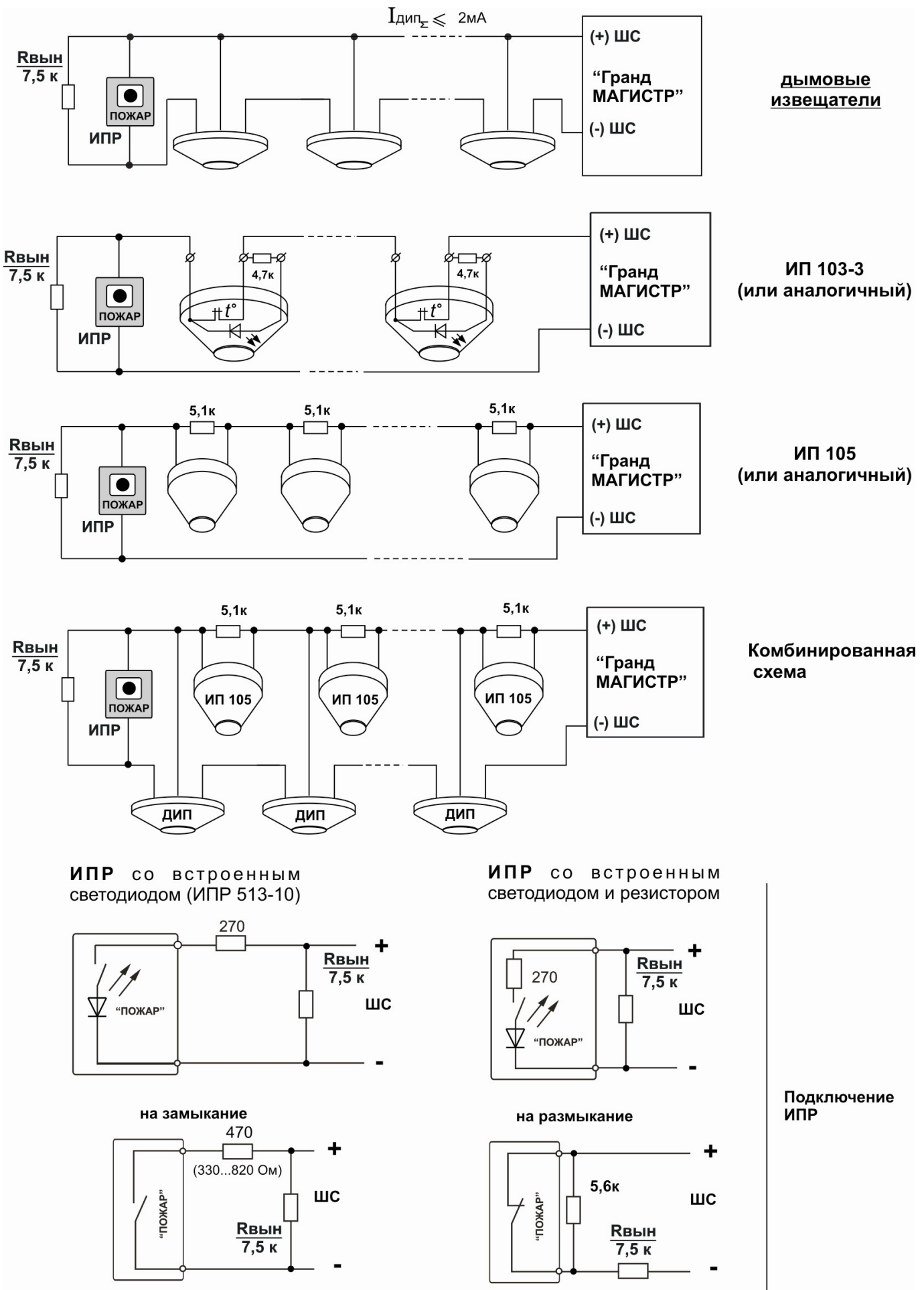
Рис. 15. Организация однопорогового шлейфа пожарной сигнализации
